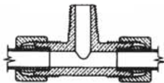
7B TEE
